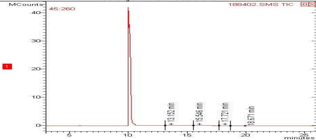
Cromatograma amostra: 10137/2013-1.0
