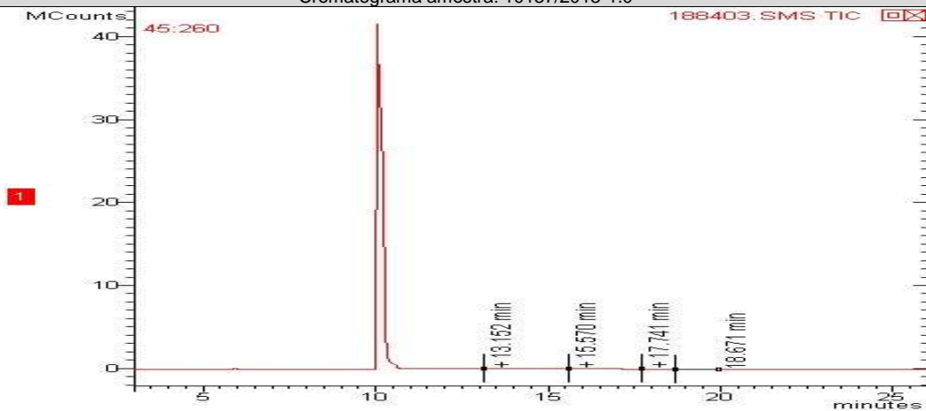
Cromatograma amostra: 10137/2013-1.0
