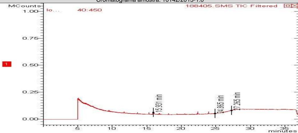
Cromatograma amostra: 10142/2013-1.0
