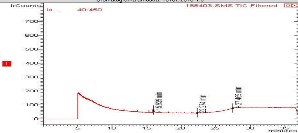
Cromatograma amostra: 10137/2013-1.0
