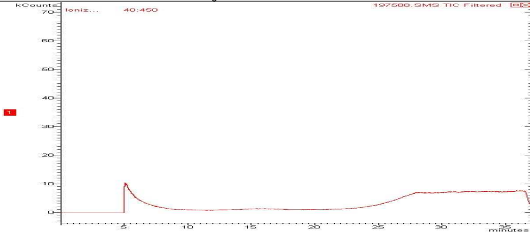
Cromatograma amostra: 18545/2013-1.0
