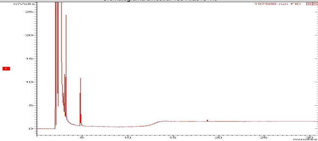
Cromatograma amostra: 18544/2013-1.0
