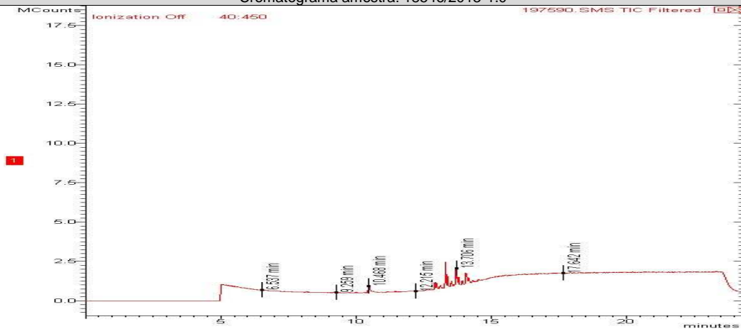
Cromatograma amostra: 18546/2013-1.0
