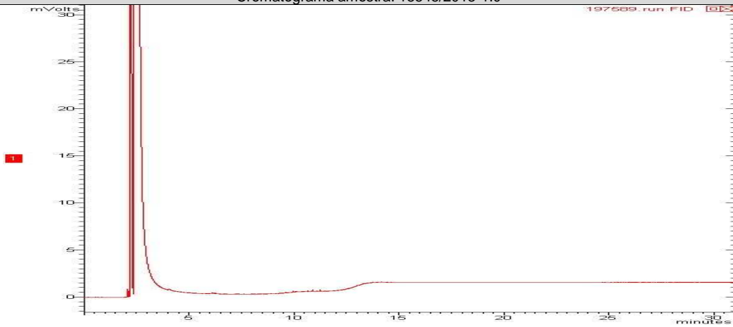
Cromatograma amostra: 18546/2013-1.0
