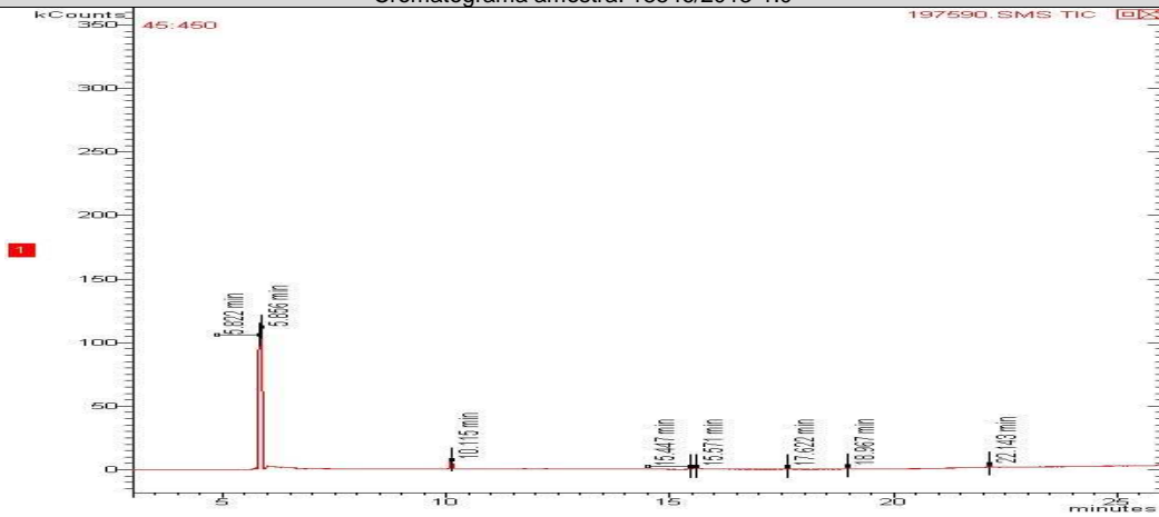
Cromatograma amostra: 18547/2013-1.0
