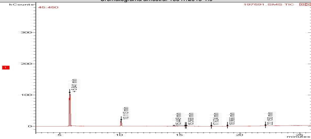
Cromatograma amostra: 18548/2013-1.0
