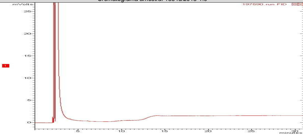
Cromatograma amostra: 18547/2013-1.0
