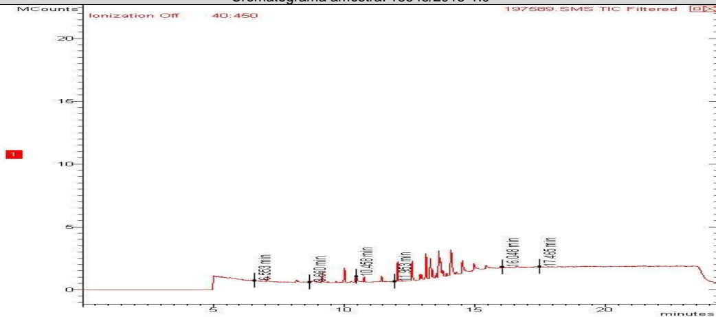
Cromatograma amostra: 18546/2013-1.0
