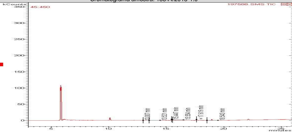
Cromatograma amostra: 18545/2013-1.0
