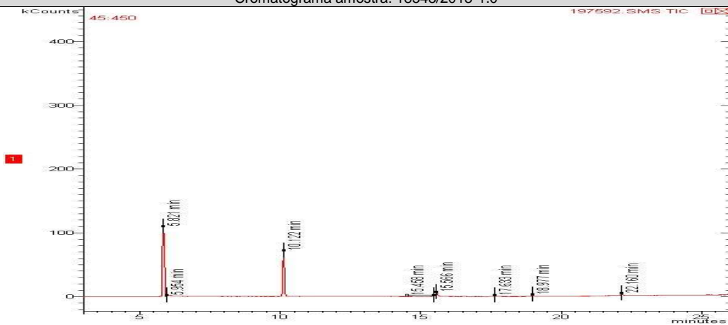
Cromatograma amostra: 18548/2013-1.0
