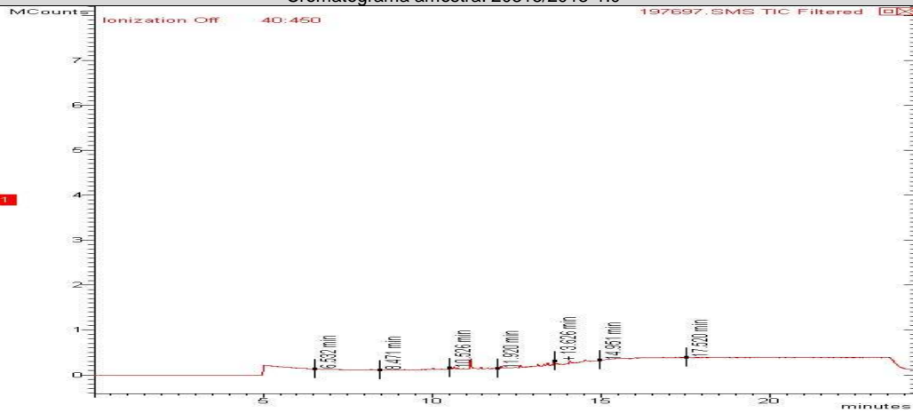
Cromatograma amostra: 20316/2013-1.0
