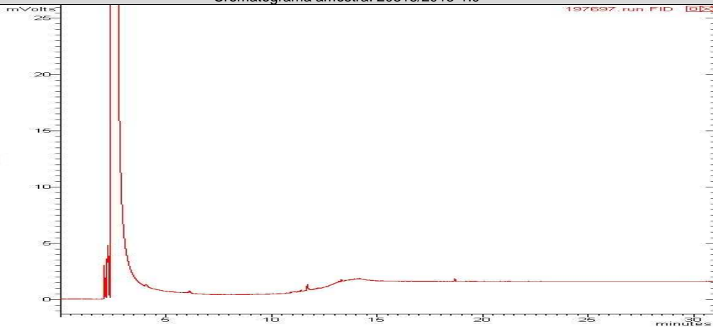
Cromatograma amostra: 20316/2013-1.0
