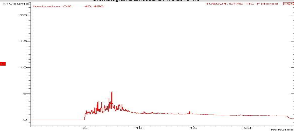
Cromatograma amostra: 21474/2013-1.0
