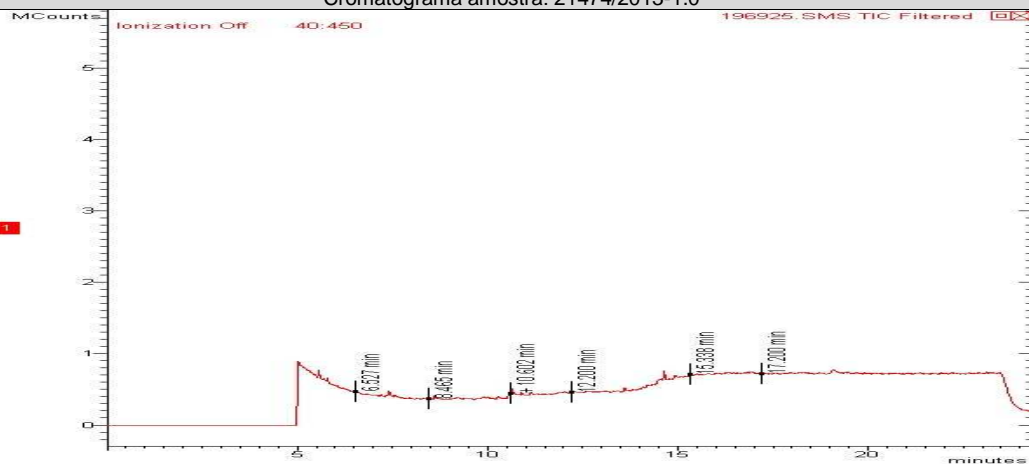
Cromatograma amostra: 21474/2013-1.0
