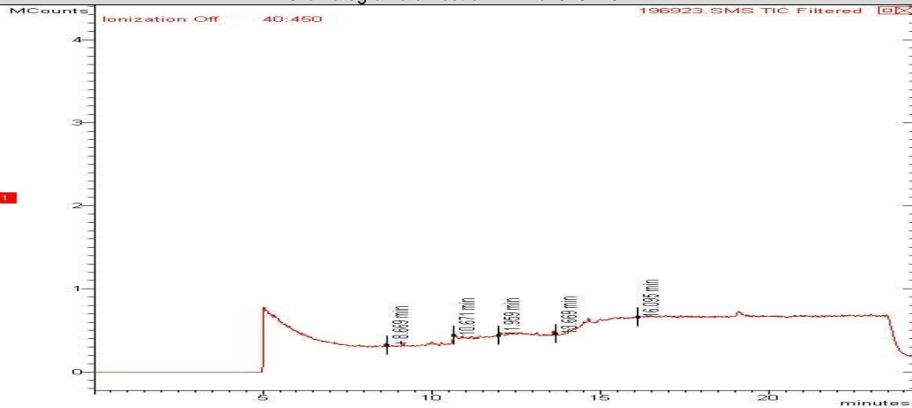
Cromatograma amostra: 21473/2013-1.0
