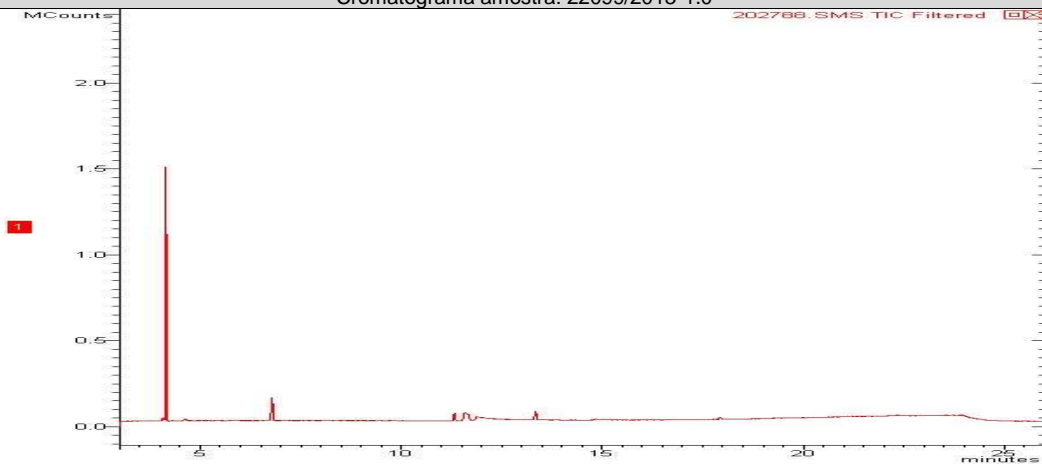
Cromatograma amostra: 22099/2013-1.0
