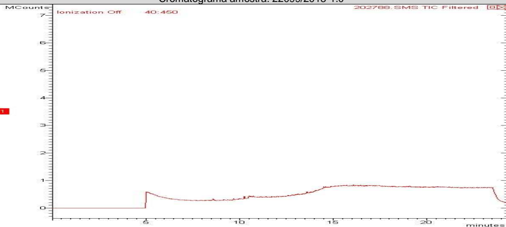
Cromatograma amostra: 22099/2013-1.0
