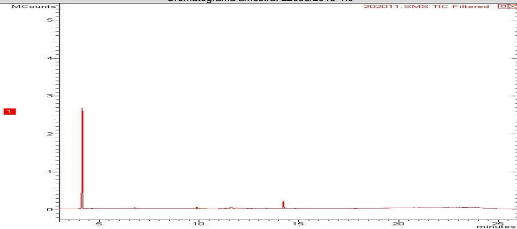
Cromatograma amostra: 22099/2013-1.0
