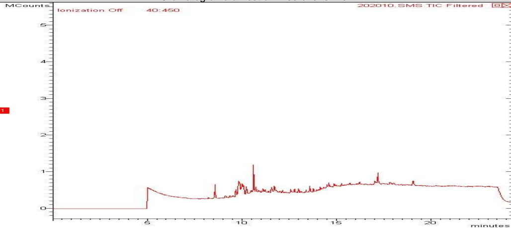
Cromatograma amostra: 22098/2013-1.0
