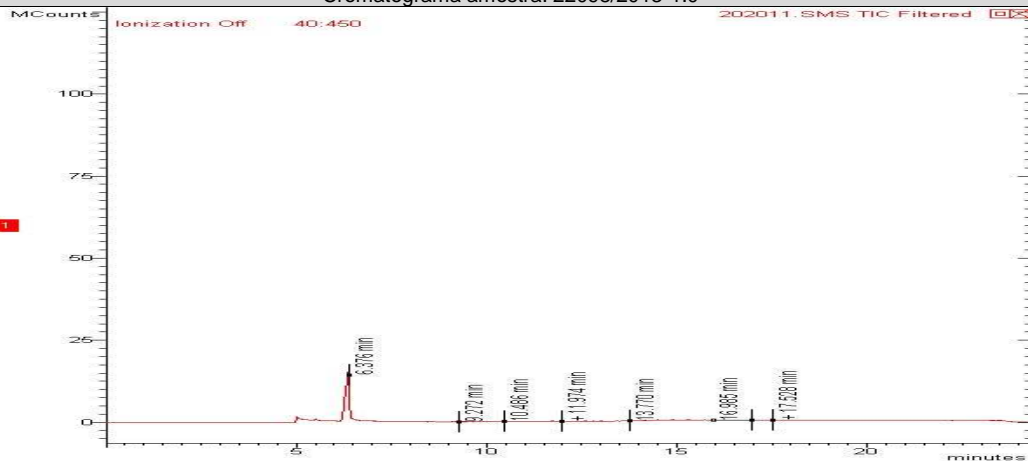
Cromatograma amostra: 22099/2013-1.0
