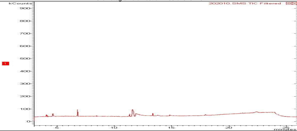
Cromatograma amostra: 22098/2013-1.0
