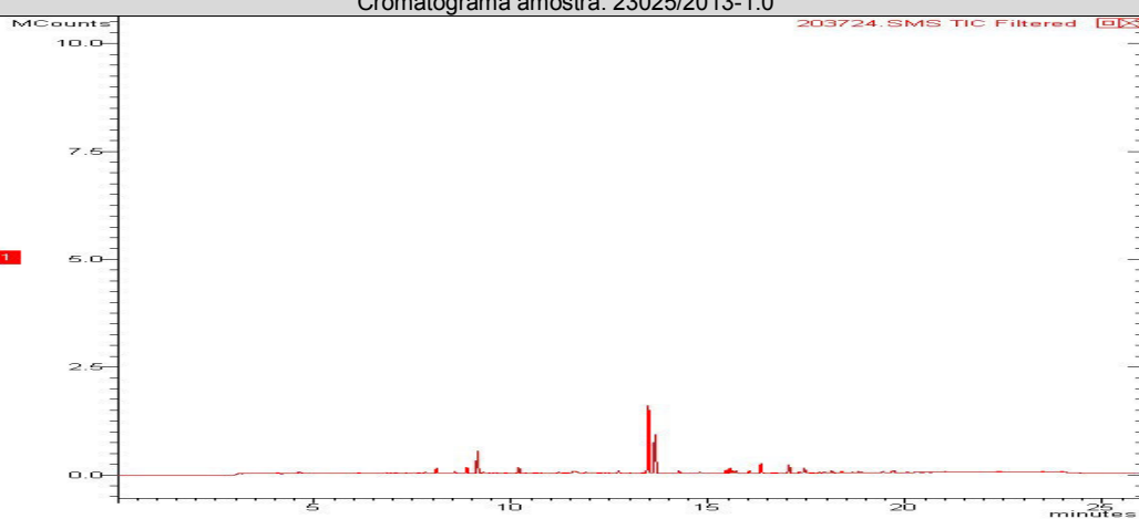
Cromatograma amostra: 23026/2013-1.0
