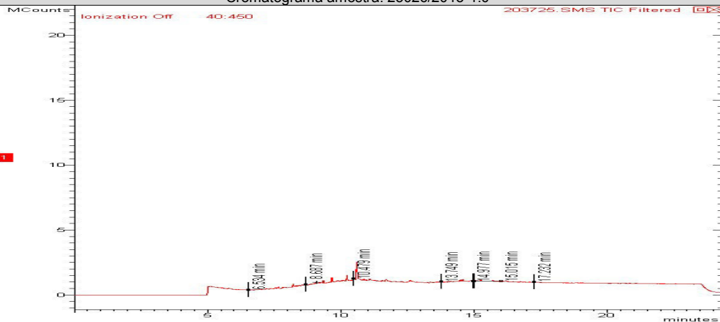
Cromatograma amostra: 23026/2013-1.0
