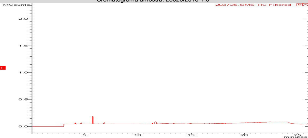
Cromatograma amostra: 23026/2013-1.0
