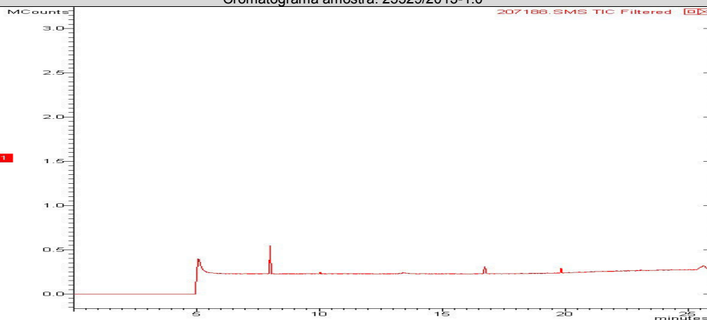
Cromatograma amostra: 25529/2013-1.0
