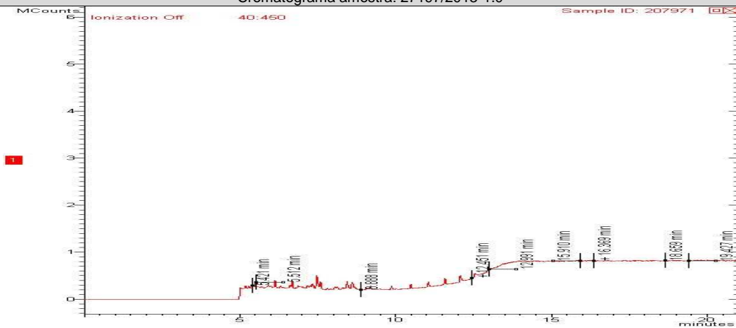
Cromatograma amostra: 27197/2013-1.0
