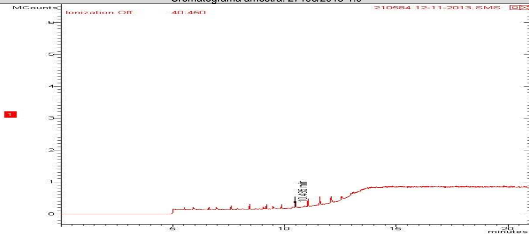
Cromatograma amostra: 27196/2013-1.0
