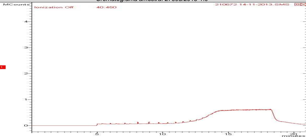
Cromatograma amostra: 27603/2013-1.0
