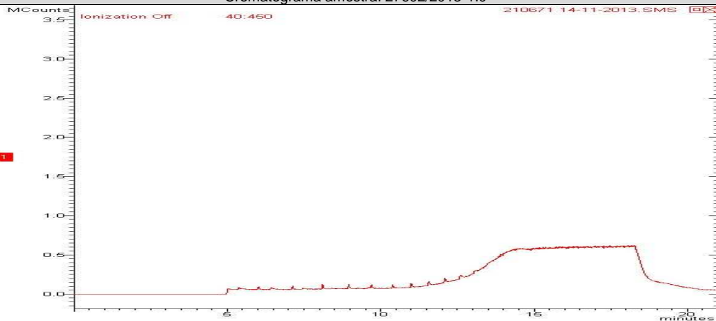
Cromatograma amostra: 27603/2013-1.0
