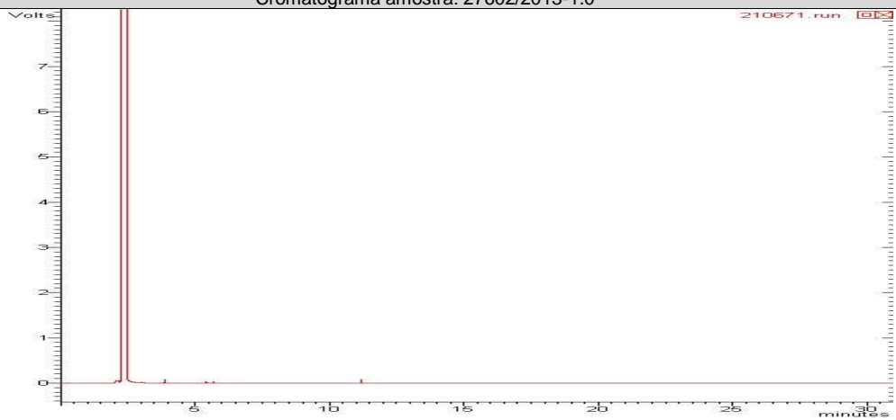
Cromatograma amostra: 27602/2013-1.0
