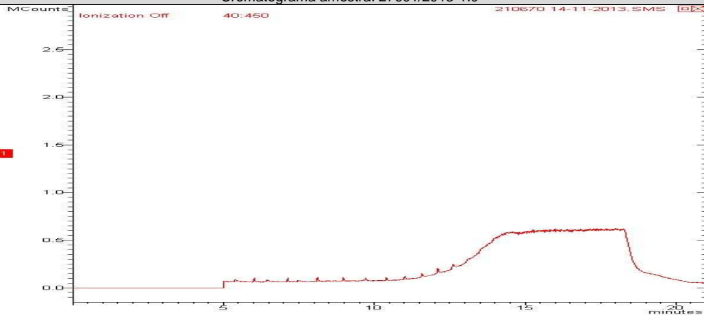
Cromatograma amostra: 27602/2013-1.0
