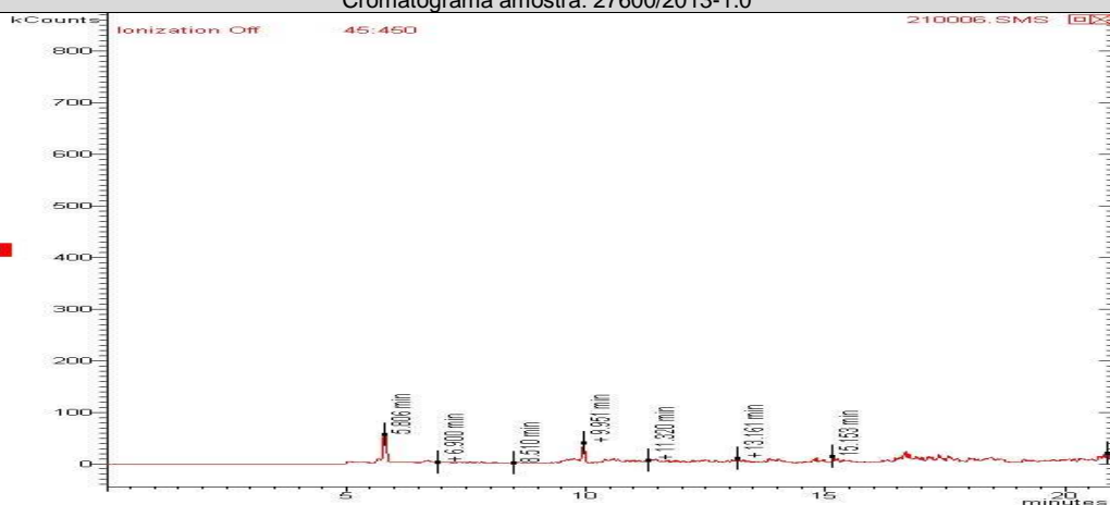
Cromatograma amostra: 27600/2013-1.0
