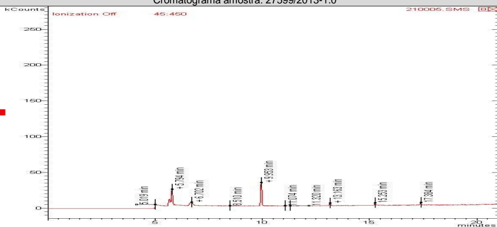
Cromatograma amostra: 27600/2013-1.0
