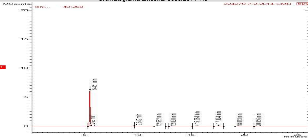
Cromatograma amostra: 3696/2014-1.0
